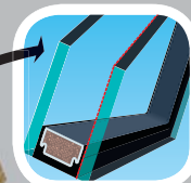
VIDRIO TERMOAISLANTE U3 Vidrio exterior templado, vidrio interior flotado con capa de baja emisividad, ensamblados en un marco aislante TGI. Cámara rellena de gas argón.
